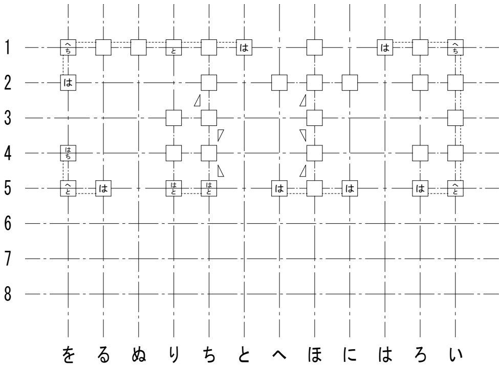
2階柱壁伏図
