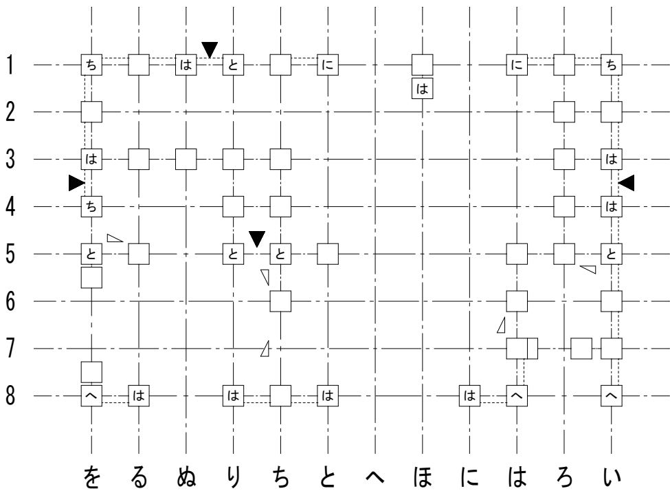
1階柱壁伏図
